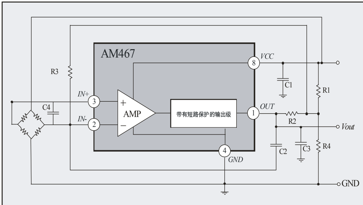
图 2：陶瓷压力传感器与 AM467 信号放大转换电路以及校准电阻网络组成的系统
